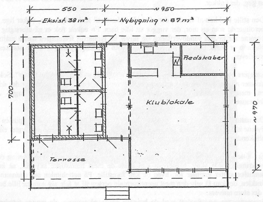
Plan 1:100 Skitseforslag_ Tegn nr 2.
